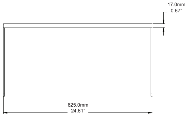
V15Y Yoke
