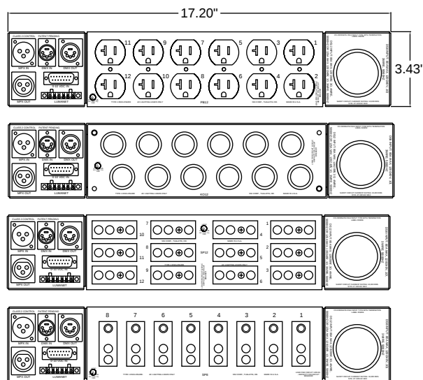
DS 8 SHOWN
