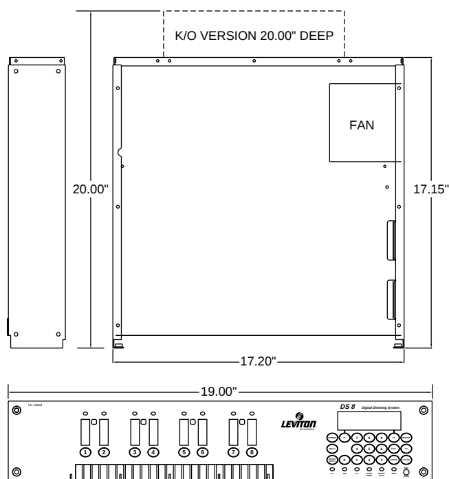
DS 8 SHOWN
