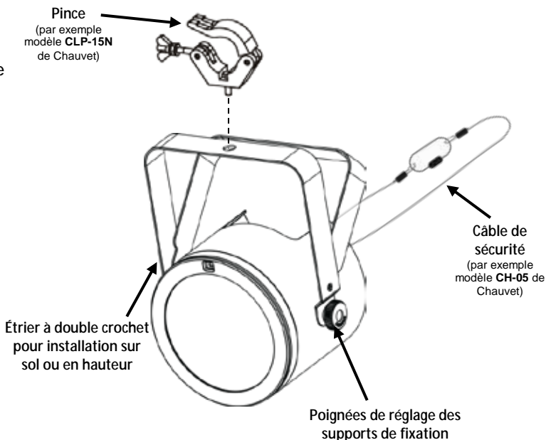
Schéma de montage
