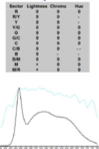
EBU : TLCI-2012 Litepanels
