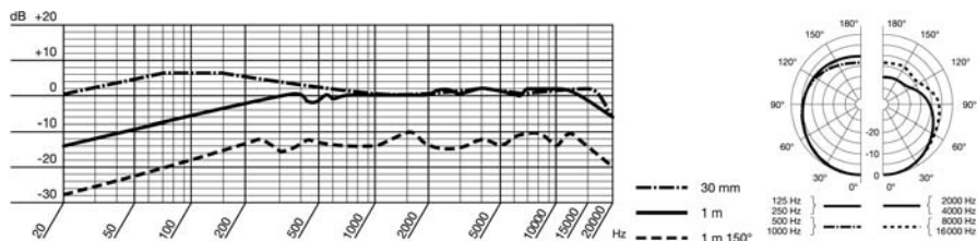
Resposta de freqüência e diagrama polar: HSC 171, HSC 271
