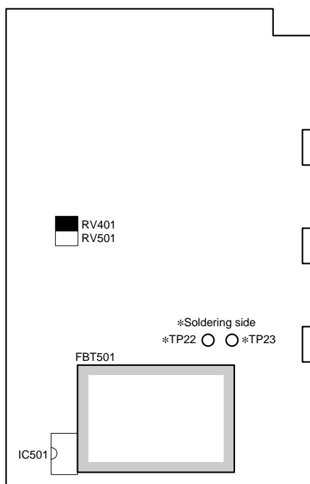
VF-70 - component side -
