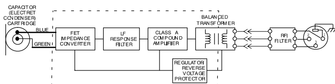
COLLEGAMENTI INTERNI FIGURA 16
