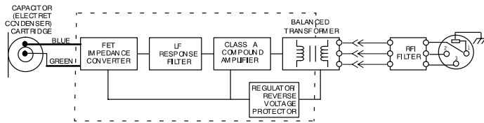
CONEXIONES INTERNAS FIGURA 12
