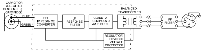
CONNEXIONS INTERNES
