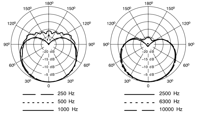
TYPISCHE POLARCHARAKTERISTIK
