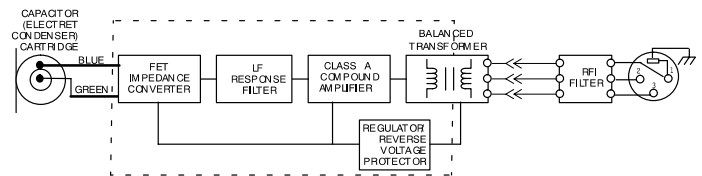
INTERNE SCHALTUNGEN
