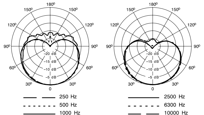
DISPERSIONES POLAR TIPICAS FIGURA 11
