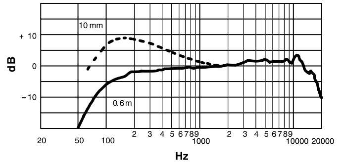
RESPUESTA DE FRECUENCIA TIPICA FIGURA 10
