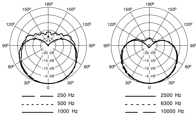
COURBES DE DIRECTIVITÉ TYPIQUES
