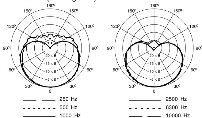
DIAGRAMMI POLARI TIPICI FIGURA 15
