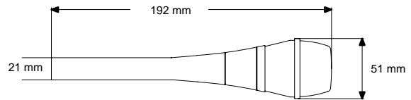
DIMENSIONES TOTALES FIGURA 5
