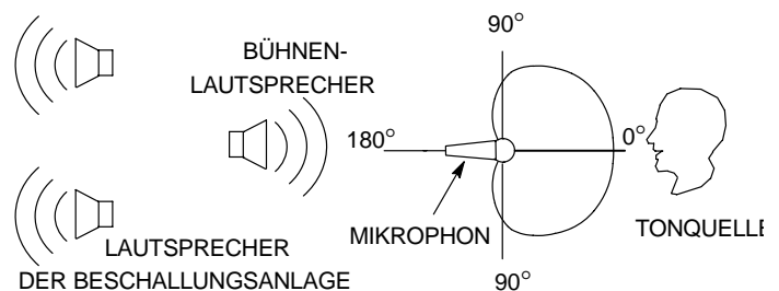
PLAZIERUNG DES NIERENMIKROFONS ABBILDUNG 5
