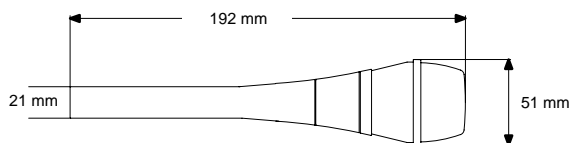
GESAMTABMESSUNGEN
