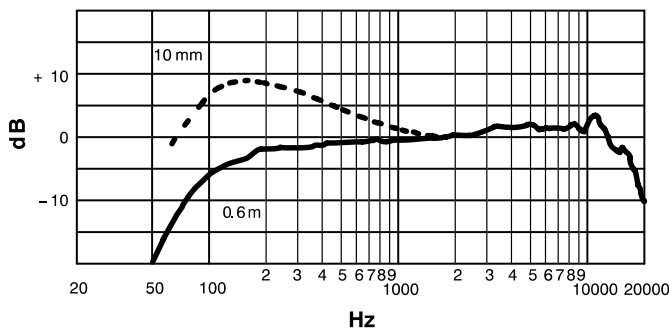
TYPISCHER FREQUENZGANG
