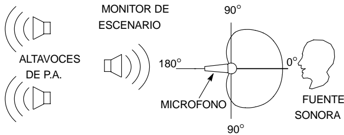
COLOCACION DEL MICROFONO DE CARDIOIDE FIGURA 9
