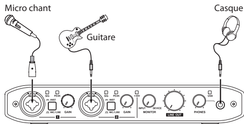
Exemple de connexion (face avant)
