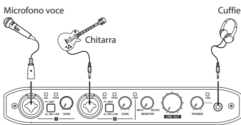
Esempio di collegamento (anteriore)
