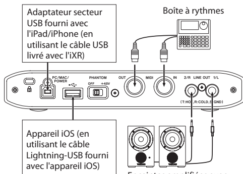
Exemple de connexion avec un appareil iOS (face arrière)
