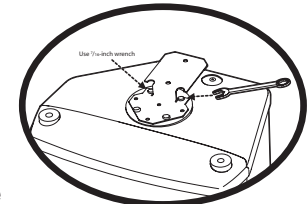
Emplacement de la Plaque du Dessus (FIGURE 2)
